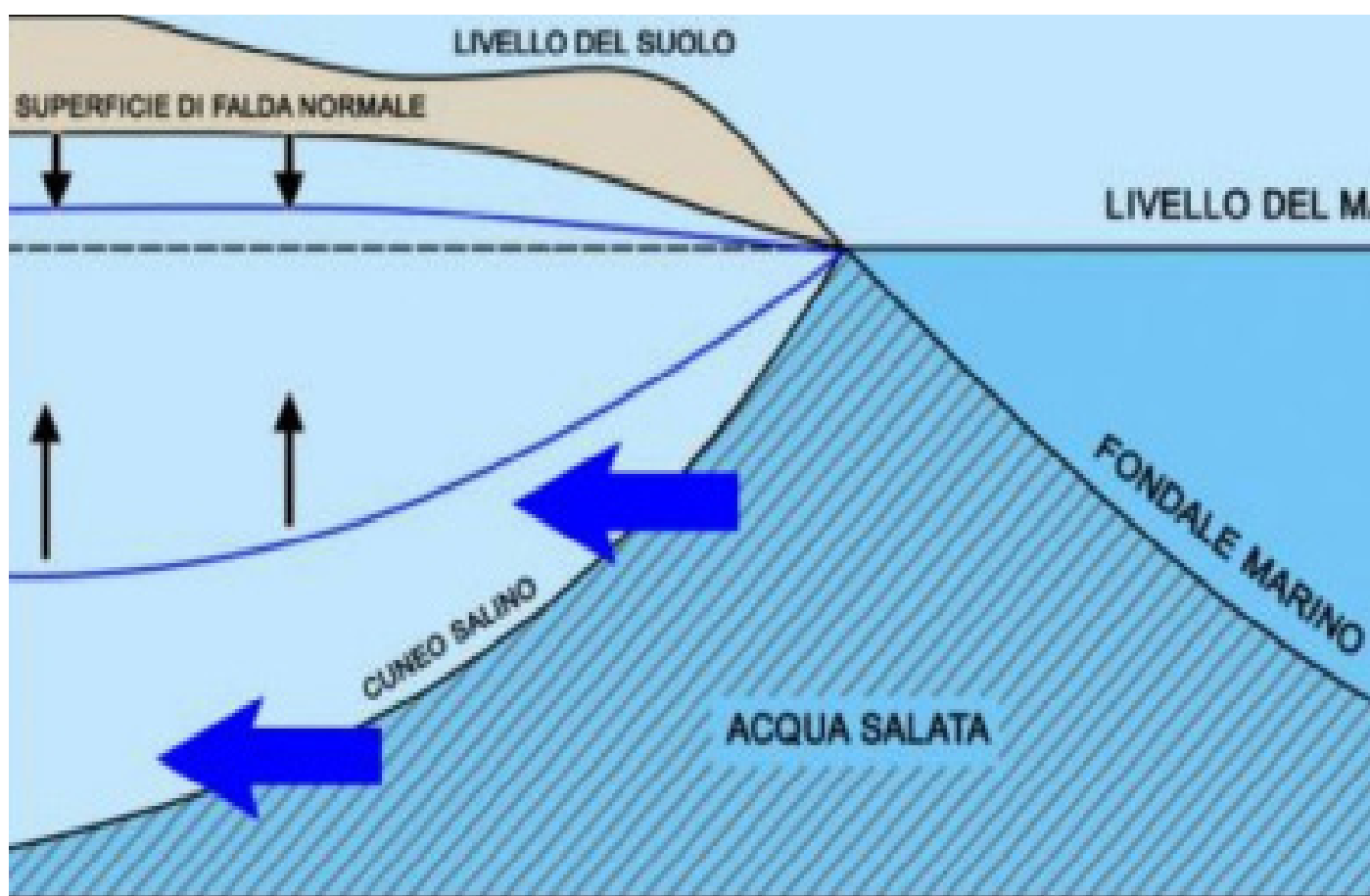
Schema del cuneo salino. Il cuneo salino è una zona di mescolamento di acqua salata e di acqua dolce che si trova sottoterra in prossimità delle foci dei fiumi. Fonte: Aprati, 2022
